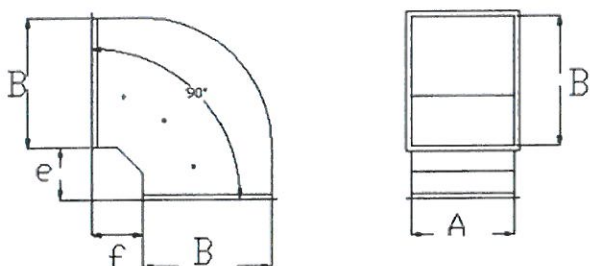
Rys. A2. Kolano symetryczne BS
