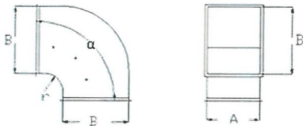
Rys. A4. Luk LP
