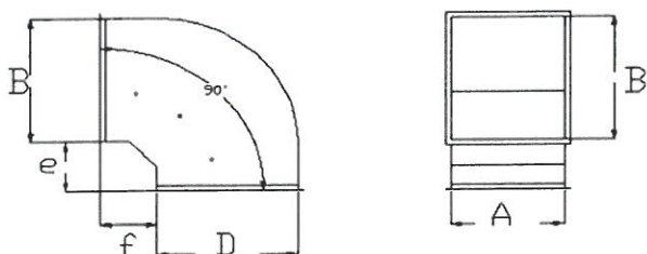
Rys. A3. Kolano asymetryczne BA
