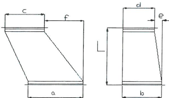
Rys. A6. Dyfuzor / redukcja asymetryczna UA
