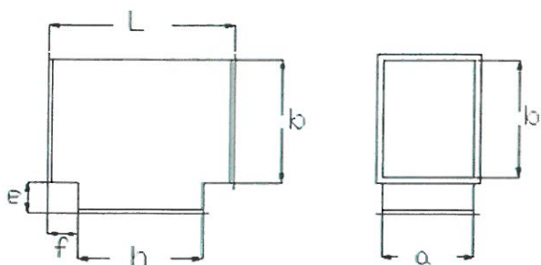
Rys. A9. Trójkąt symetryczny TRS
