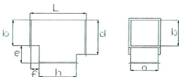
Rys. A10. Trójkąt asymetryczny TRA
