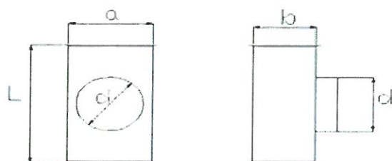
Rys. A11. Trójkąt prostokątny z odejściem okrągłym TRO
