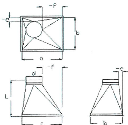
Rys. A8. Redukcja kołowo - prostokątna asymetryczna RA
