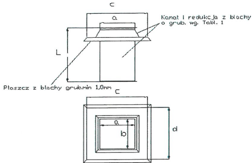
Rys. A16. Podstawa dachowa PD-PII
